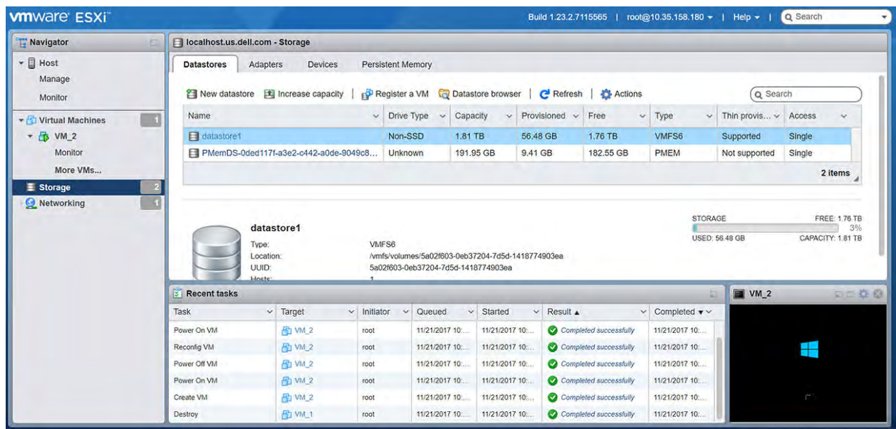
Figure 34. Datastores
